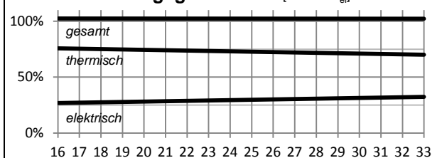
Wirkungsgradkurven [% zu kW el ]
