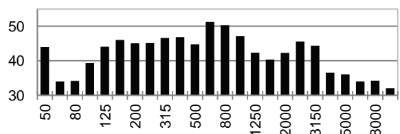
Schalldruckpegelkurve [dB(A) zu Hz] 5)
