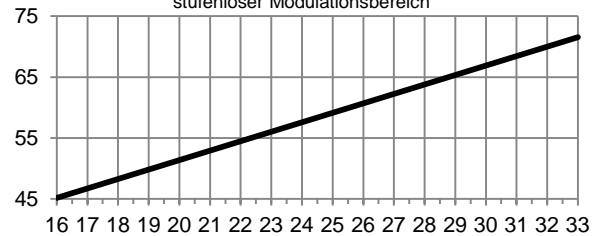
Leistungskurve [kW th zu kW el ] stufenloser Modulationsbereich
